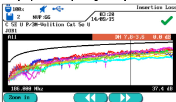
Wykres parametru Insertion Loss
